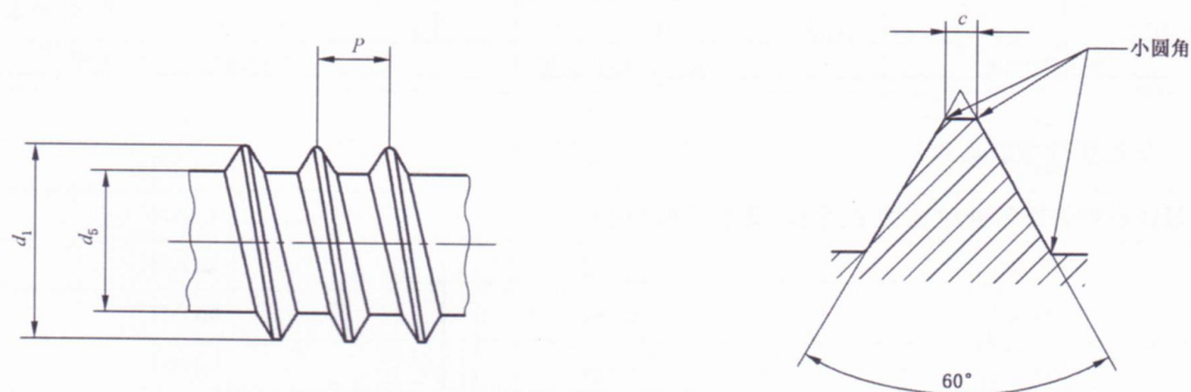
图 7 HC 型接骨螺钉螺纹
