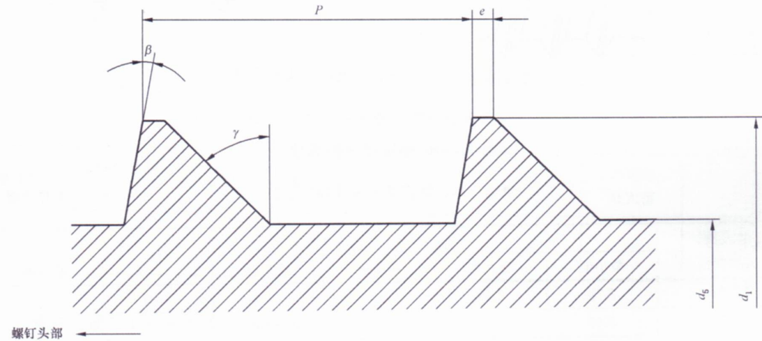
图 9 HD 型接骨螺钉螺纹
