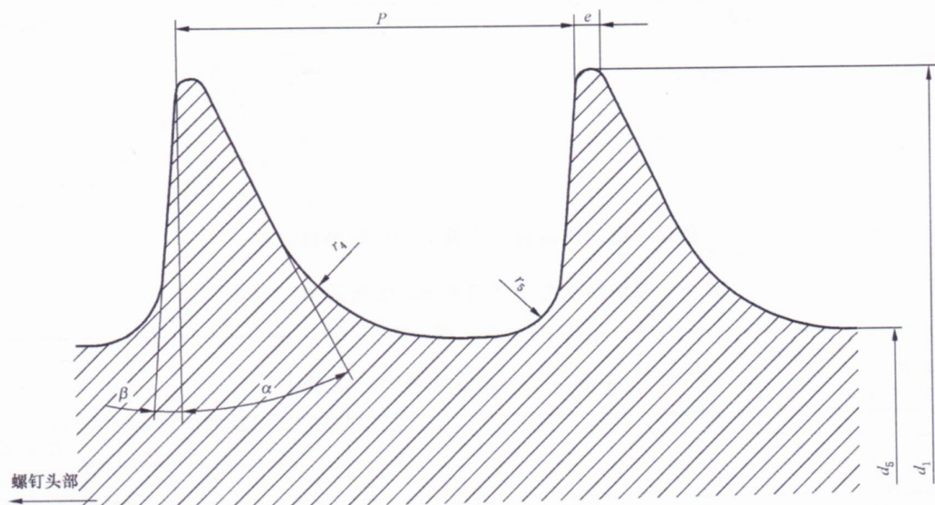
图 4 深螺纹(HB 型)
