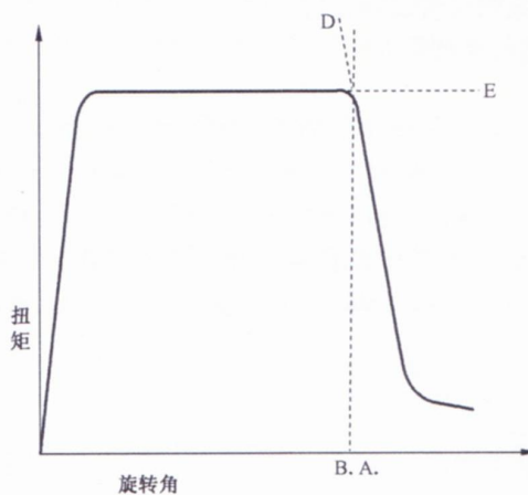
图 D.1 典型的扭矩-扭转角曲线图
