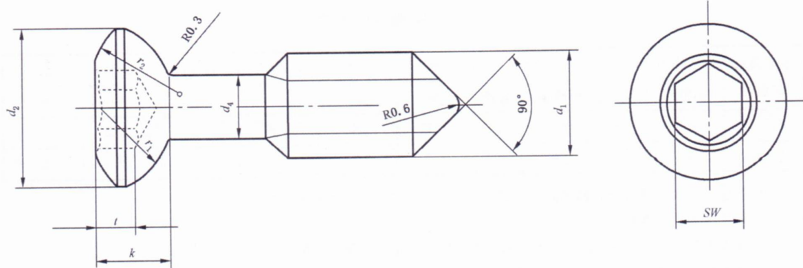
图 3 HB 型接骨螺钉
