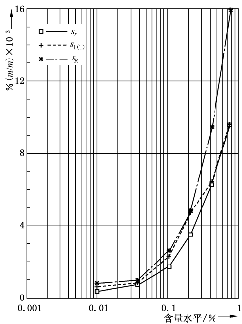
图 D.3 钢中的钒含量——重复性标准差 s_r 、时间不同的中间精密度标准差 s_{I(T)} 和再现性标准差 s_R 与钒成分含量水平的关系
