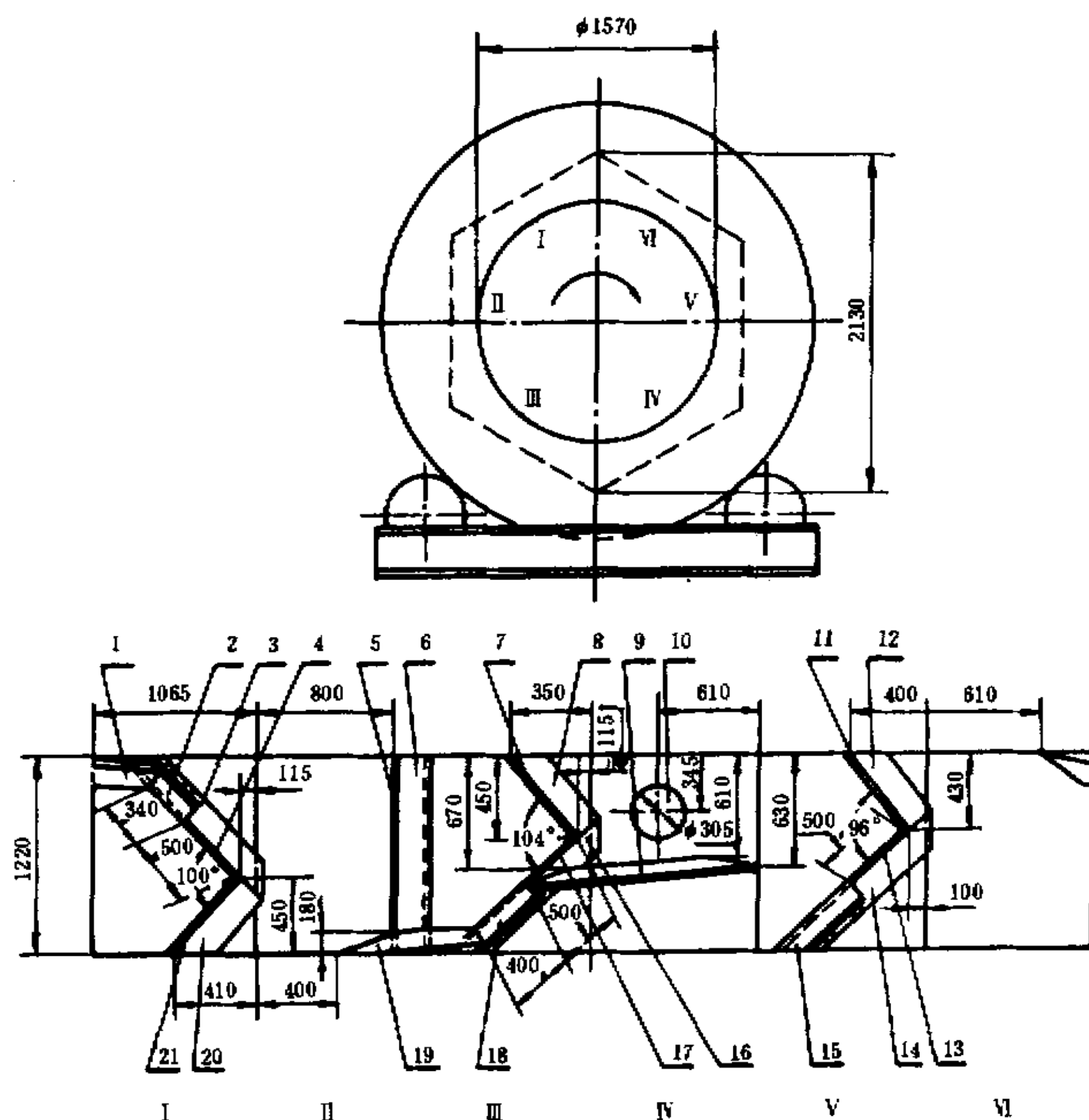
图 1 2130 型六角滚筒试验机结构尺寸示意图
