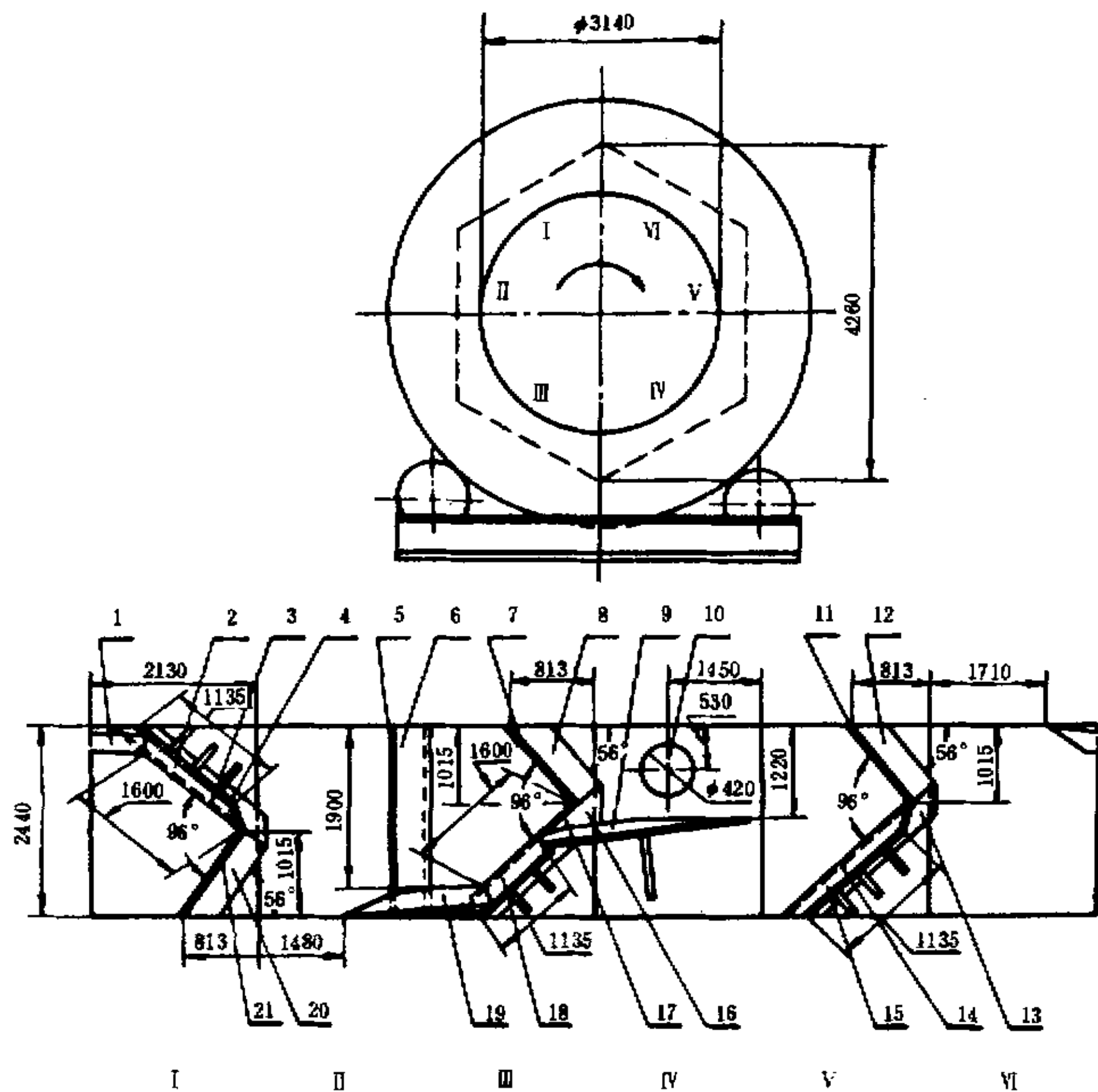
图 2 4260 型六角滚筒试验机结构尺寸示意图 表 2 4260 型六角滚筒试验机构件材料、尺寸
