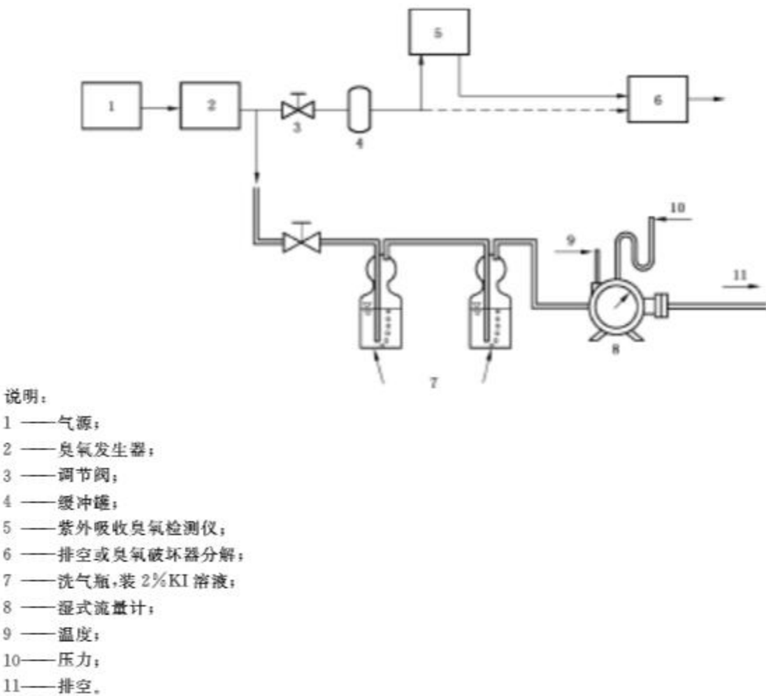
图 B.3 校准系统简图
