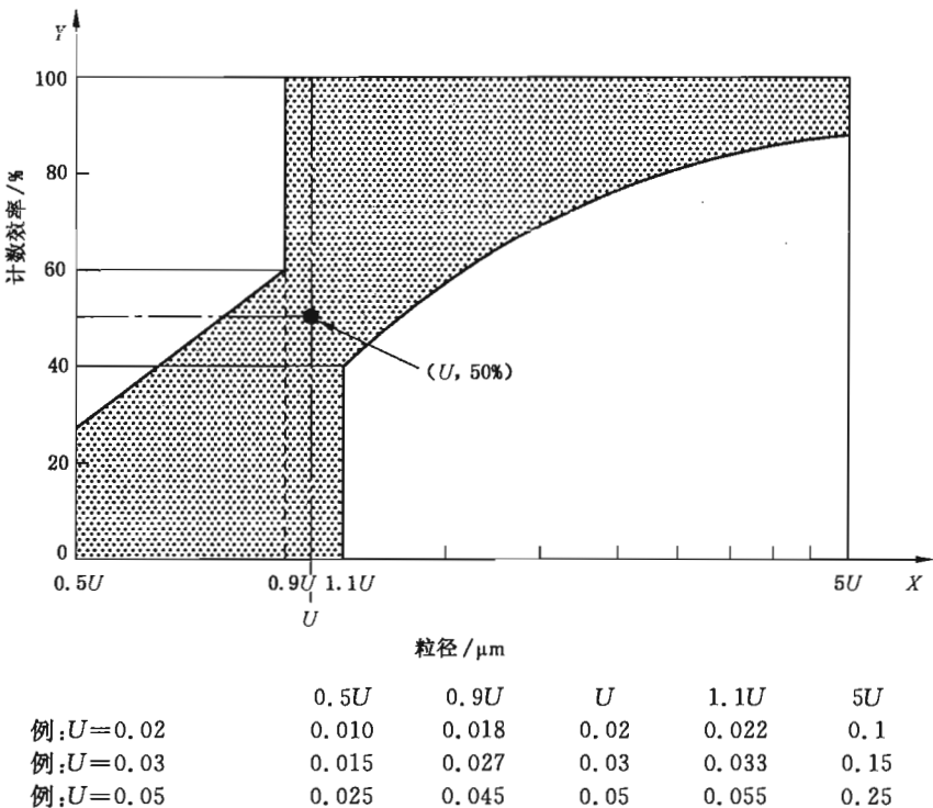
图 B.1 所选仪器计数效率达标区
