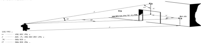
图 20 观察角、最大观察距离、偏移和偏移角示意
