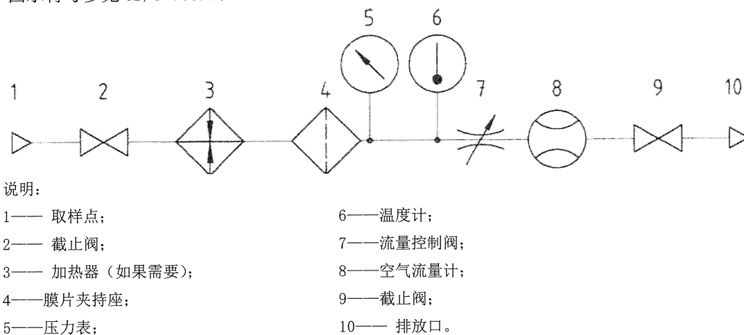
图 1 重量法试验设备布置图
