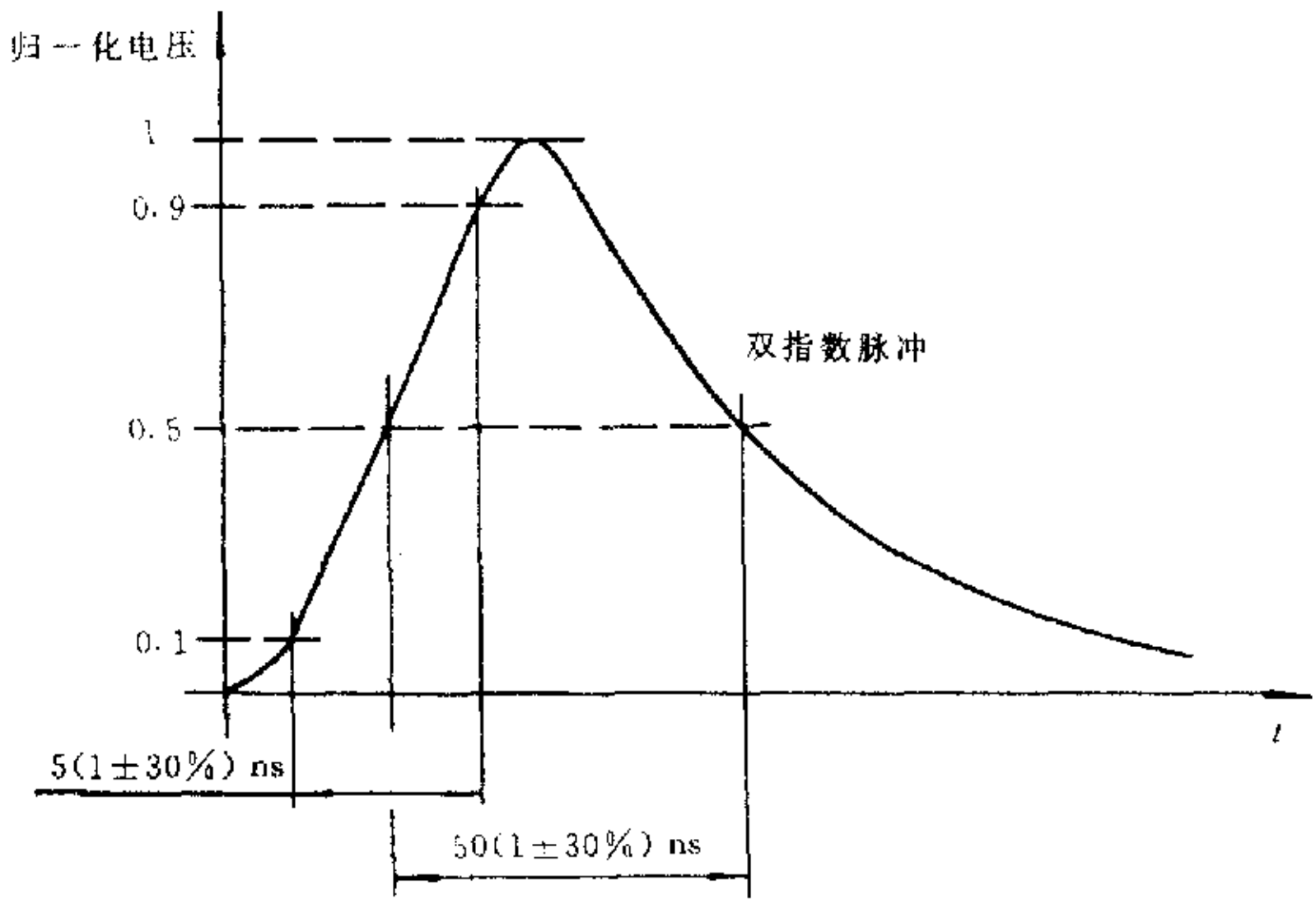
图 3 接 50 \Omega 负载时单个脉冲的波形
