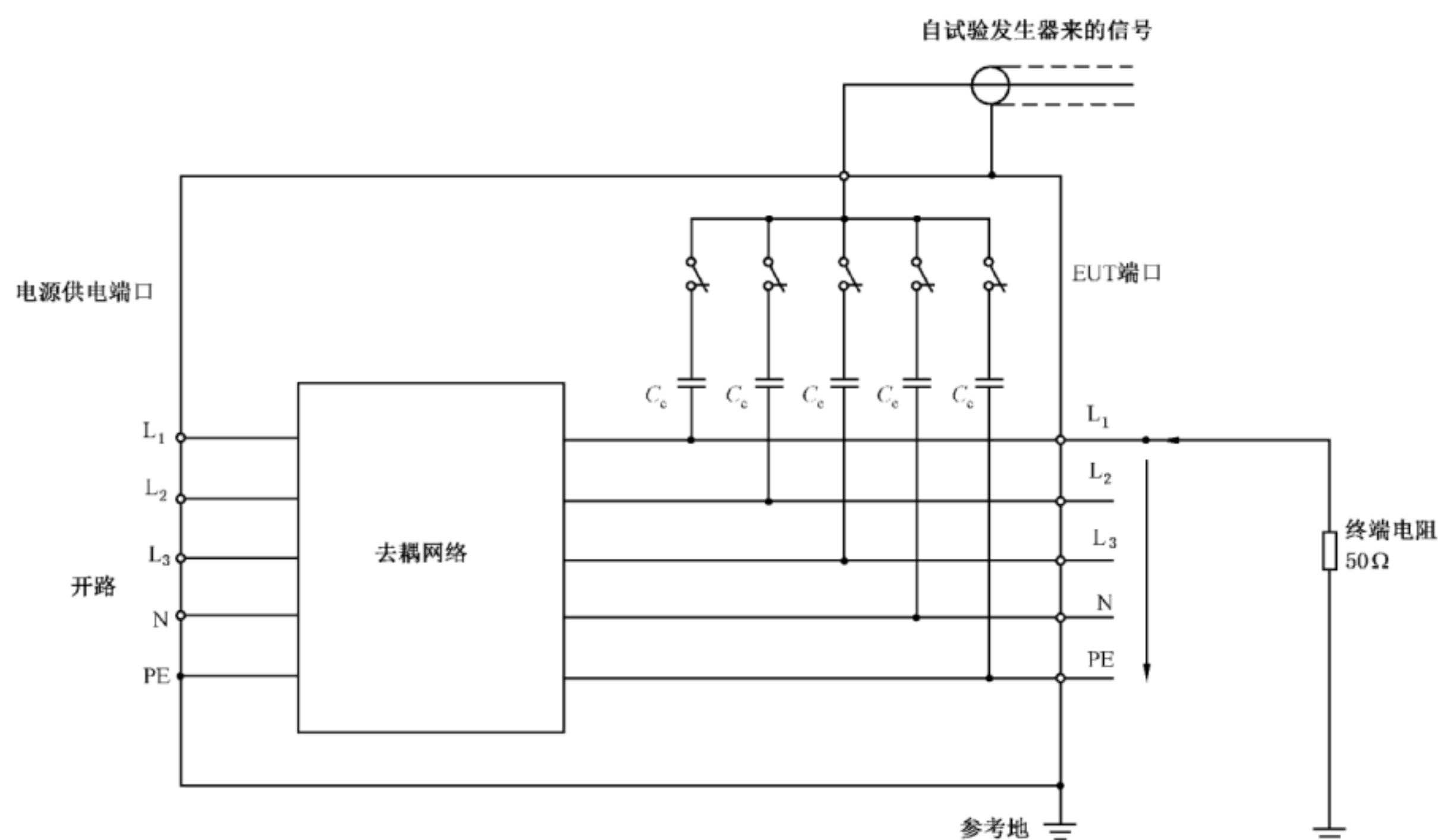
图 5 耦合/去耦网络输出端波形校准
