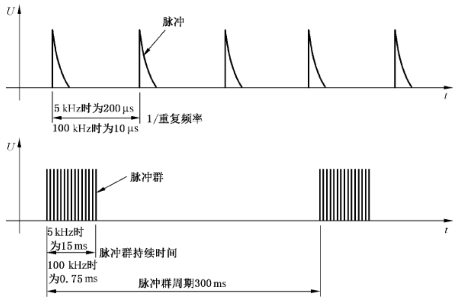
图 2 电快速瞬变脉冲群概略图
