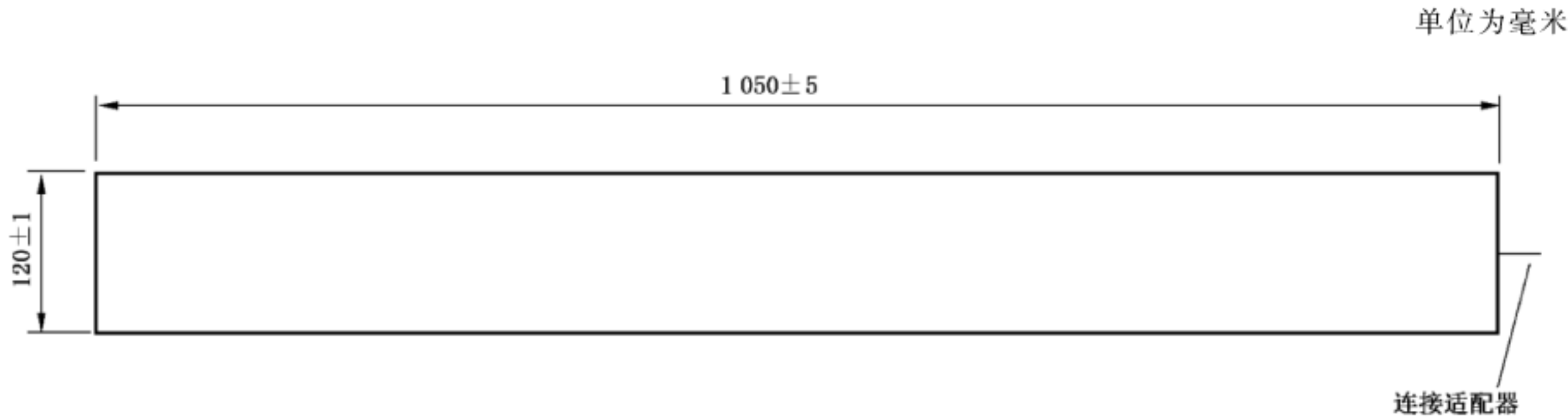
图7 用于耦合夹校准的感应板
