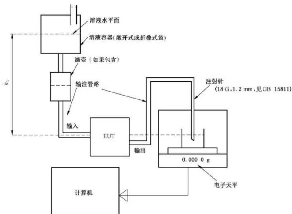
a) 容量式输液泵和容量式输液控制器试验装置
