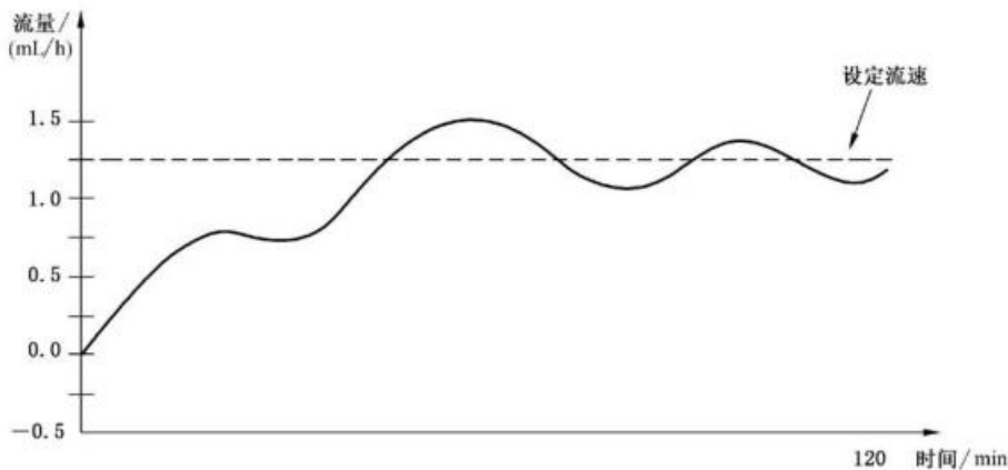
图 201.103 根据试验周期的最初 2 h 期间采集的数据作成的上升曲线图
