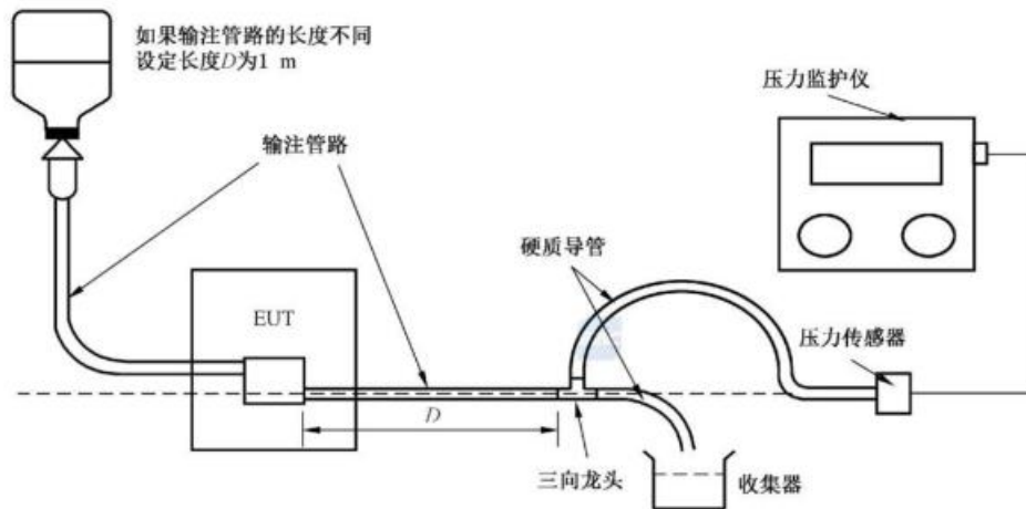
图 201.110 确定阻塞报警阈值和丸剂量的试验装置
