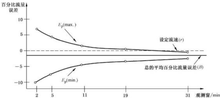
图 201.105 根据输注管路更换间隔最后一个小时采集的数据作成的喇叭曲线图
