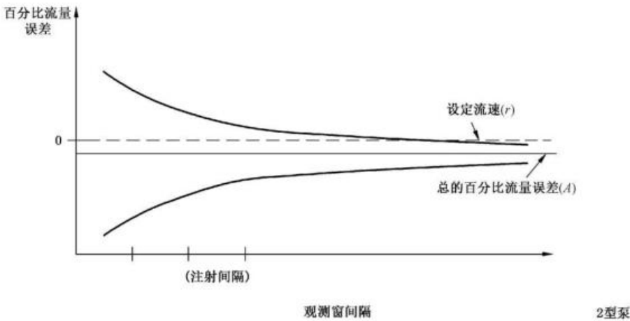
图 201.109 稳定周期结束时根据数据得出的半连续泵喇叭曲线图
