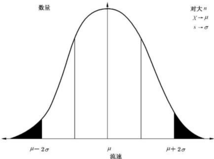
图 AA.6 原始变量 X 的分布图
