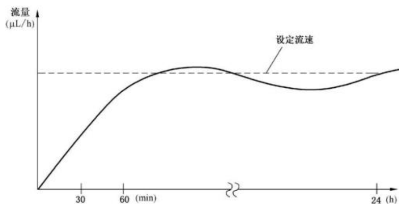
图 201.106 稳定周期阶段的上升图
