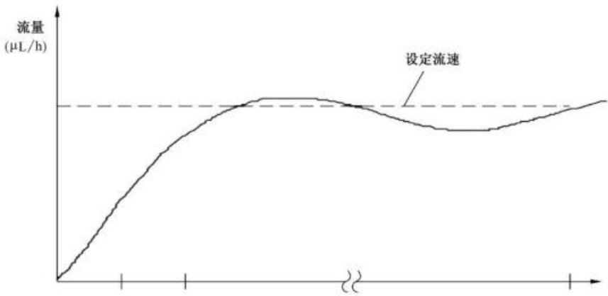
图 201.108 稳定周期中半连续输出泵的上升曲线图
