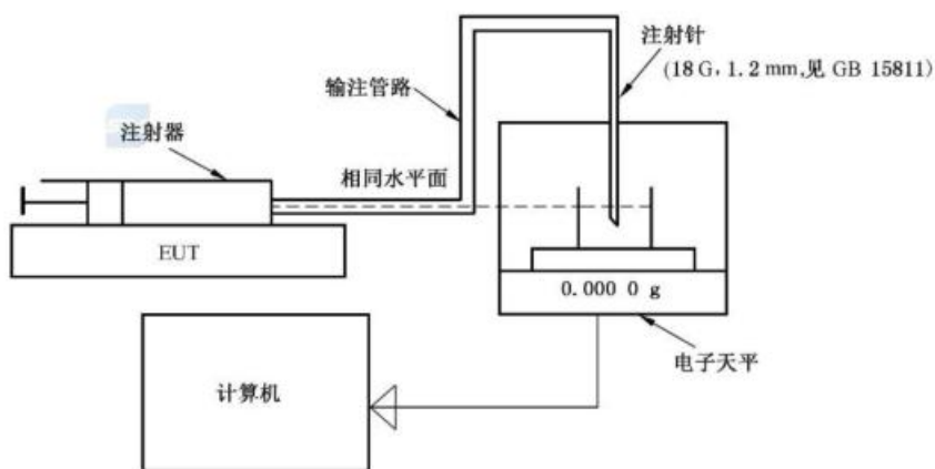
b) 注射/容器泵试验装置
