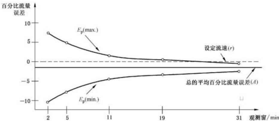
图 201.104 根据试验周期第 2 个小时期间采集的数据作成的喇叭曲线图
