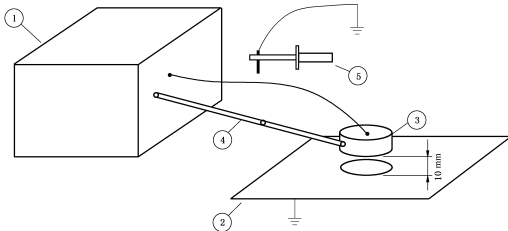
图 201.102 测试探头
