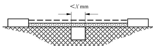
图 22 爬电距离和电气间隙——示例 1
