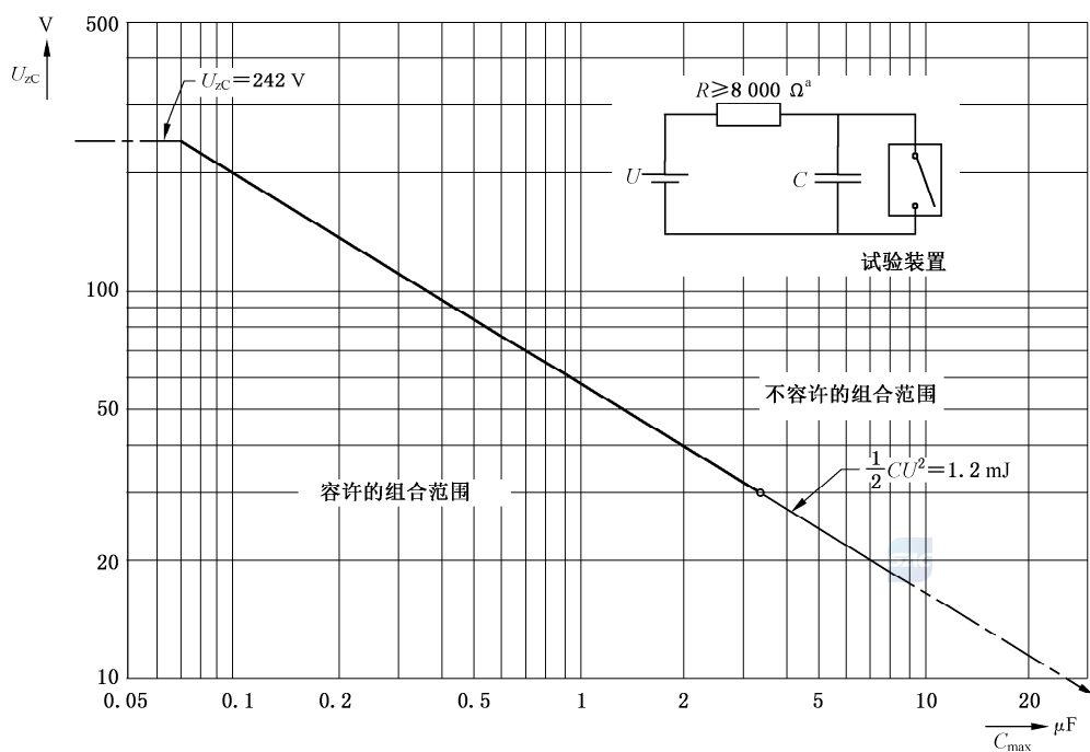
图 G.2 在乙醚蒸气和空气混合成的最易燃气体中电容电路上测得的 最大容许电压 U_{x\text{C}} 和电容 C_{\text{max}} 的函数关系
