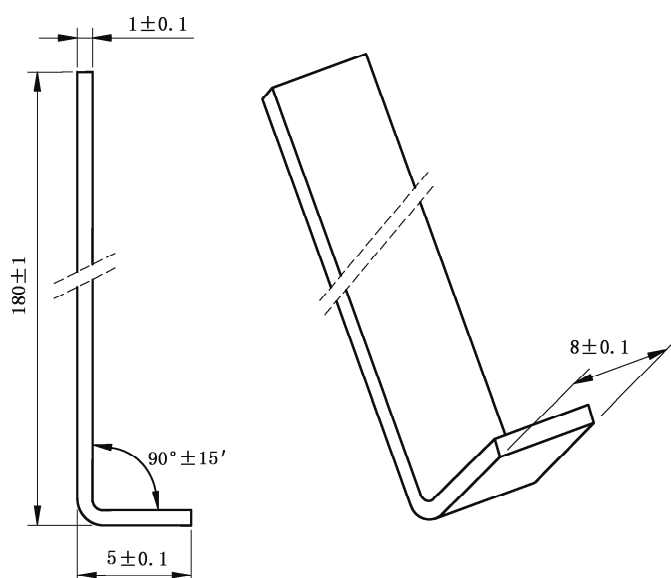
图7 试验钩(见 5.9.2.2)
