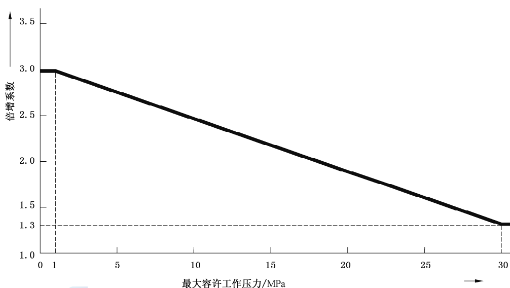
图 32 水压试验压力与最大容许工作压力的比例关系（见 9.7.5）
