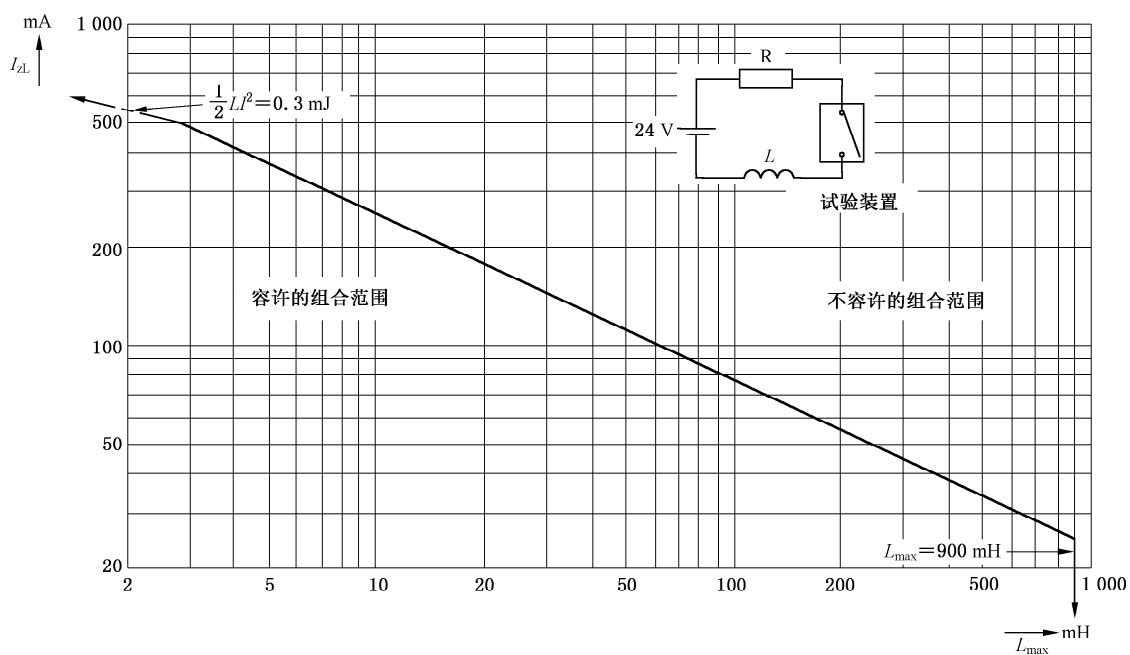
图 G.3 在乙醚蒸气和空气混合成的最易燃气体中电感电路上测得的 最大容许电流 I_{z\text{L}} 和电感 L_{\text{max}} 的函数关系
