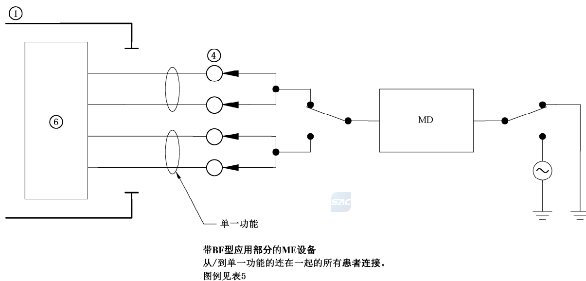
图 E.2 BF 型应用部分
