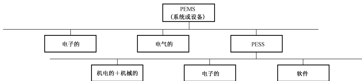
b) 较为简单系统示例
