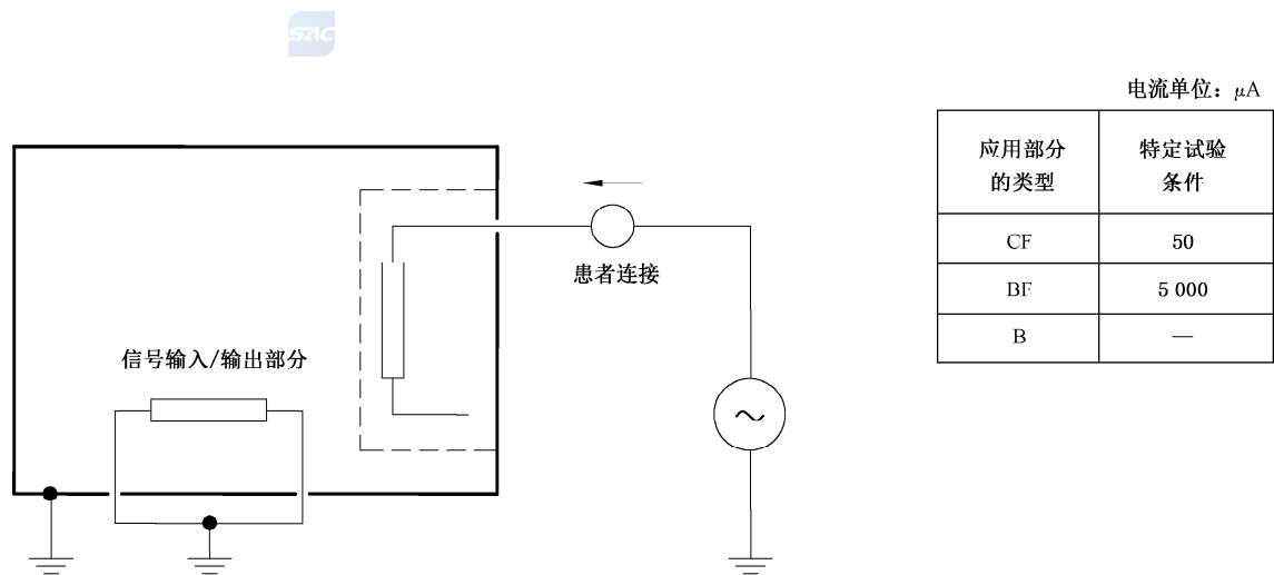
图 K.1 带有由绝缘材料制成的外壳的 ME 设备 (简化的图 15) [见 8.7.4.7 a)]
