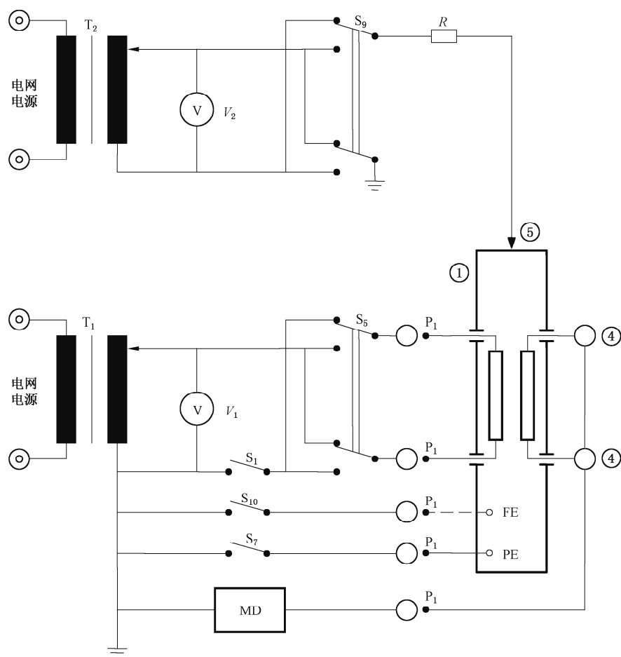
图例见表 5。 说明： 闭合 S_1 (如果是 I 类 ME 设备, 还要闭合 S_7 ) , 在 S_5 、 S_9 和 S_{10} 的开、闭位置进行所有可能组合的情况下进行测量。 对于 II 类 ME 设备, 不使用保护接地连接和 S_7 。 采用图 F.1 的测量供电电路的图例。
