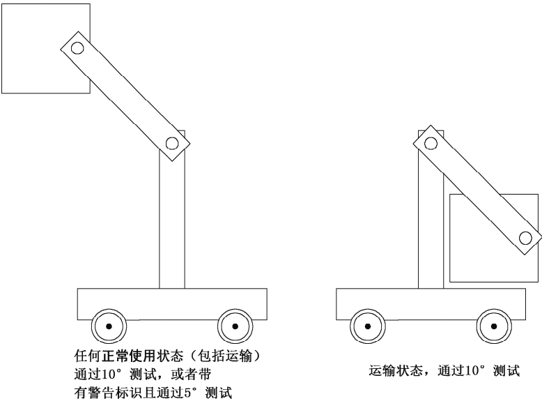
图 A.16 不稳定性试验条件
