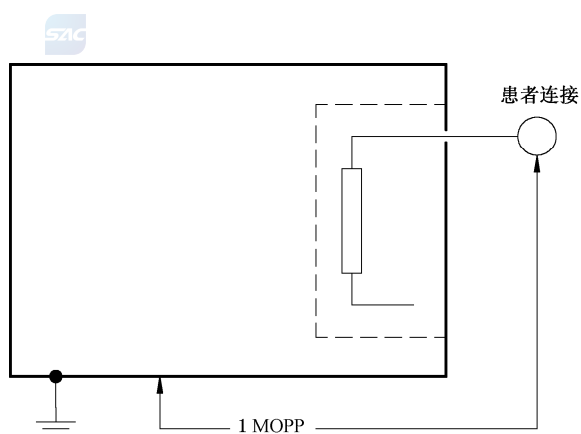
图 J.6 绝缘示例 6
