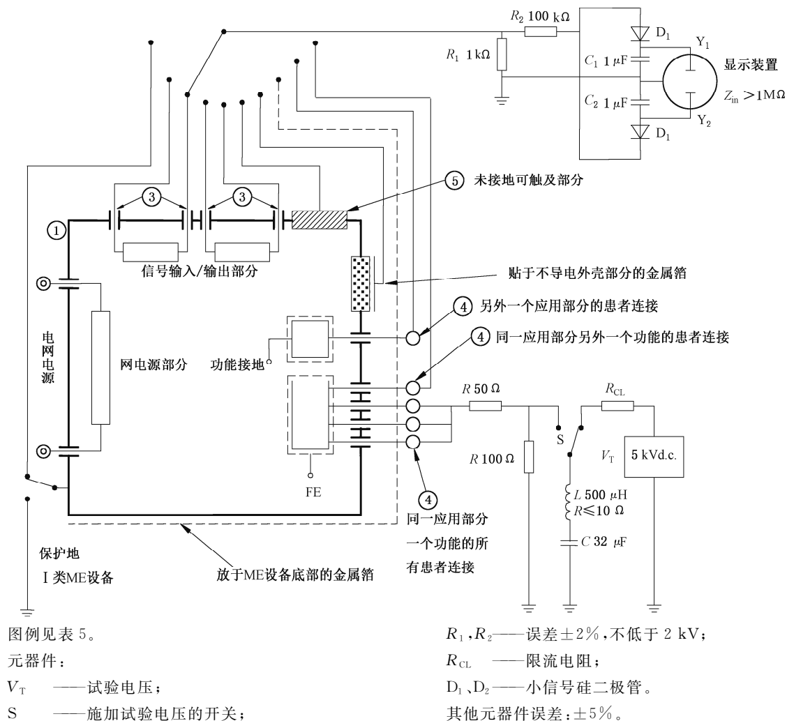
图 9 试验电压施加于桥接的防除颤应用部分的患者连接(见 8.5.5.1)
