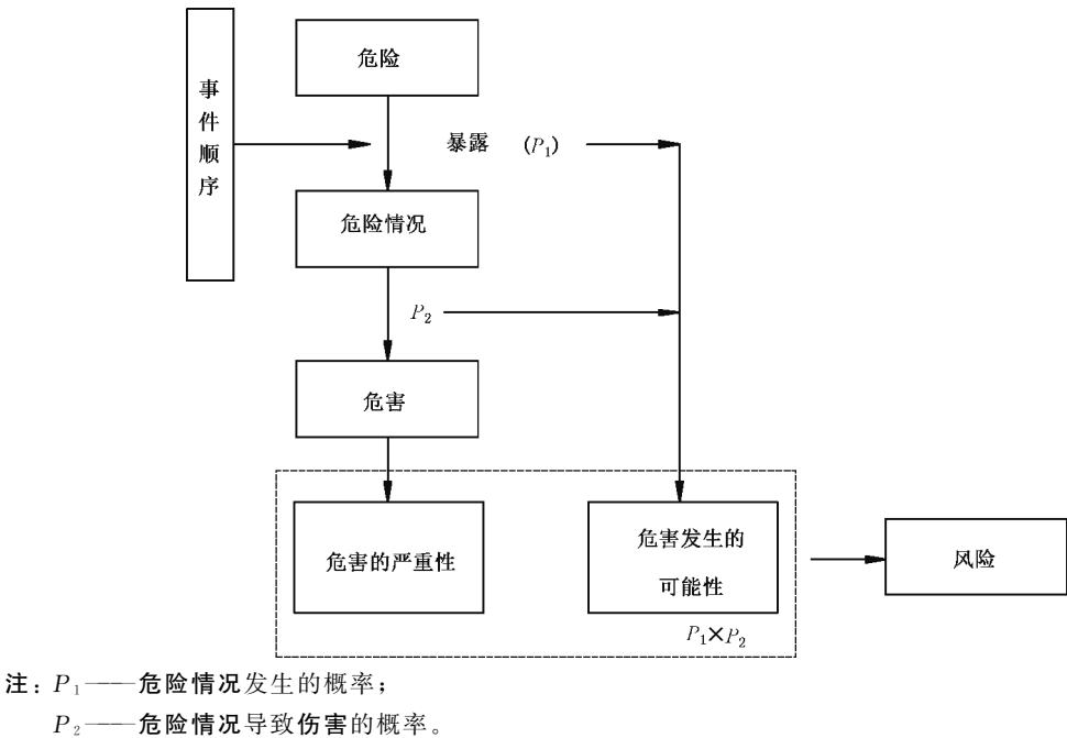
图 A.8 危害、续发事件、风险情况和伤害的关系图
