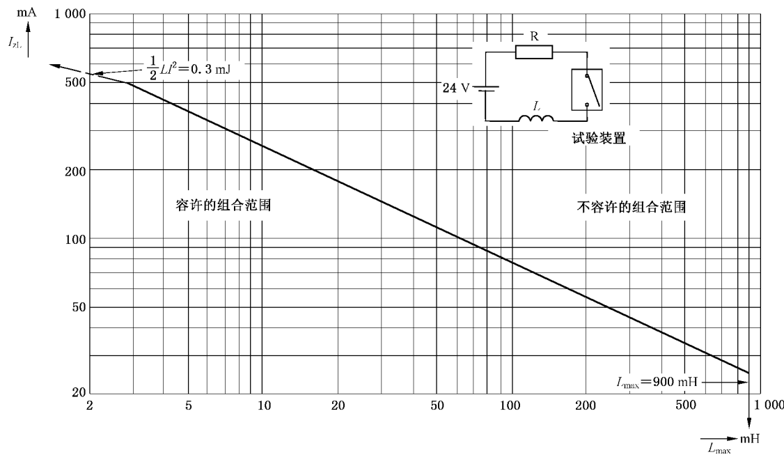
图 G.3 在乙醚蒸气和空气混合成的最易燃气体中电感电路上测得的 最大容许电流 I_{xL} 和电感 L_{max} 的函数关系
