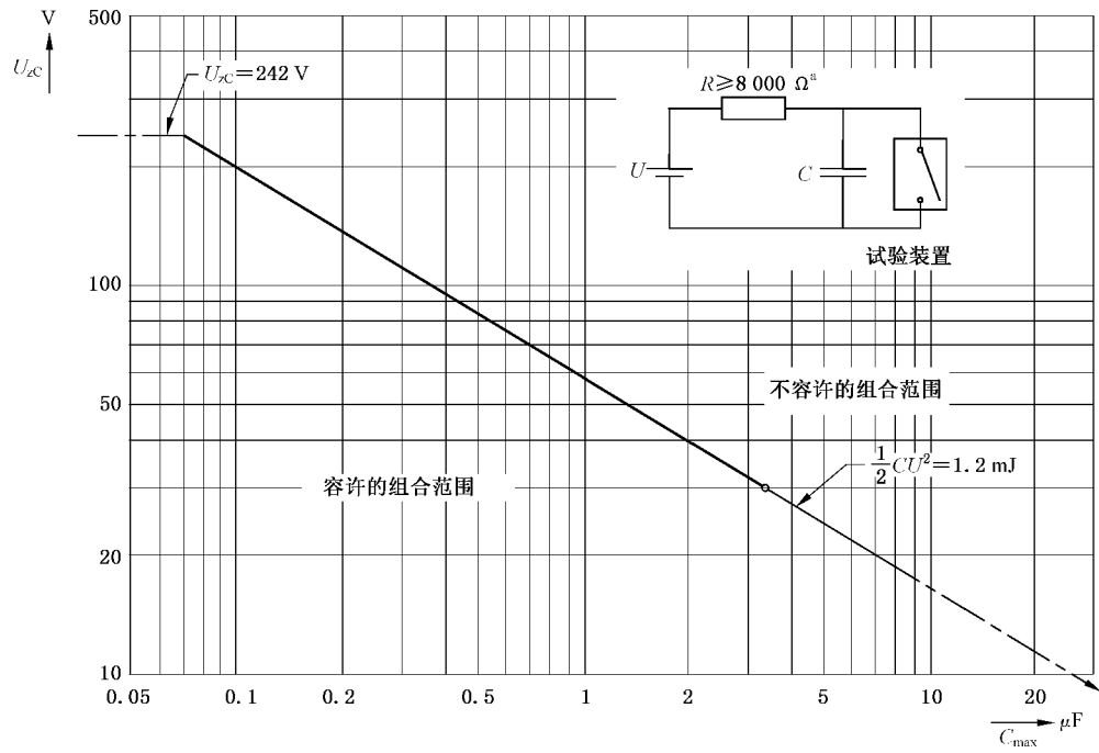
图 G.2 在乙醚蒸气和空气混合成的最易燃气体中电容电路上测得的 最大容许电压 U_{xc} 和电容 C_{max} 的函数关系
