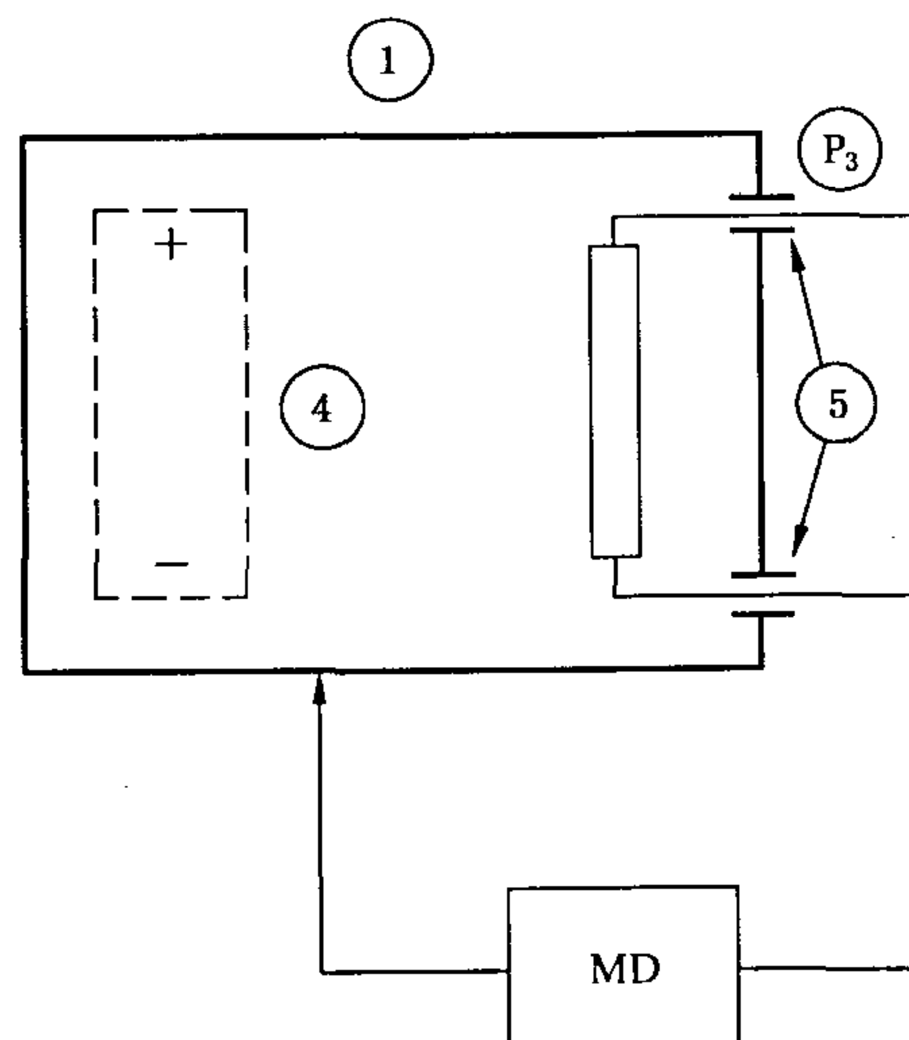
图 22 由信号输入部分或信号输出部分上的外来电压引起的从应用部分至地的患者漏电流的测量电路 对 II 类设备时不使用保护接地连接和 S_7 采用图 10 的测量供电电路的图例[见 19.4 h)]
