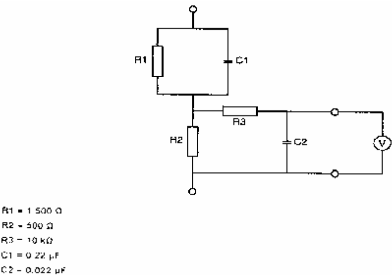
图 A.1 频率小于或等于 1MHz 的交流和直流测量电路
