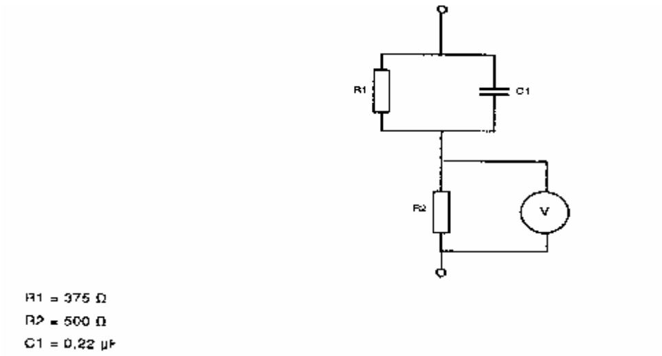
图 A.4 潮湿接触电流测量电路
