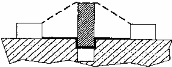
例 8 通过未粘接接缝的爬电距离小于越过挡板的爬电距离。 电气间隙是越过挡板顶部最短直达空间距离。
