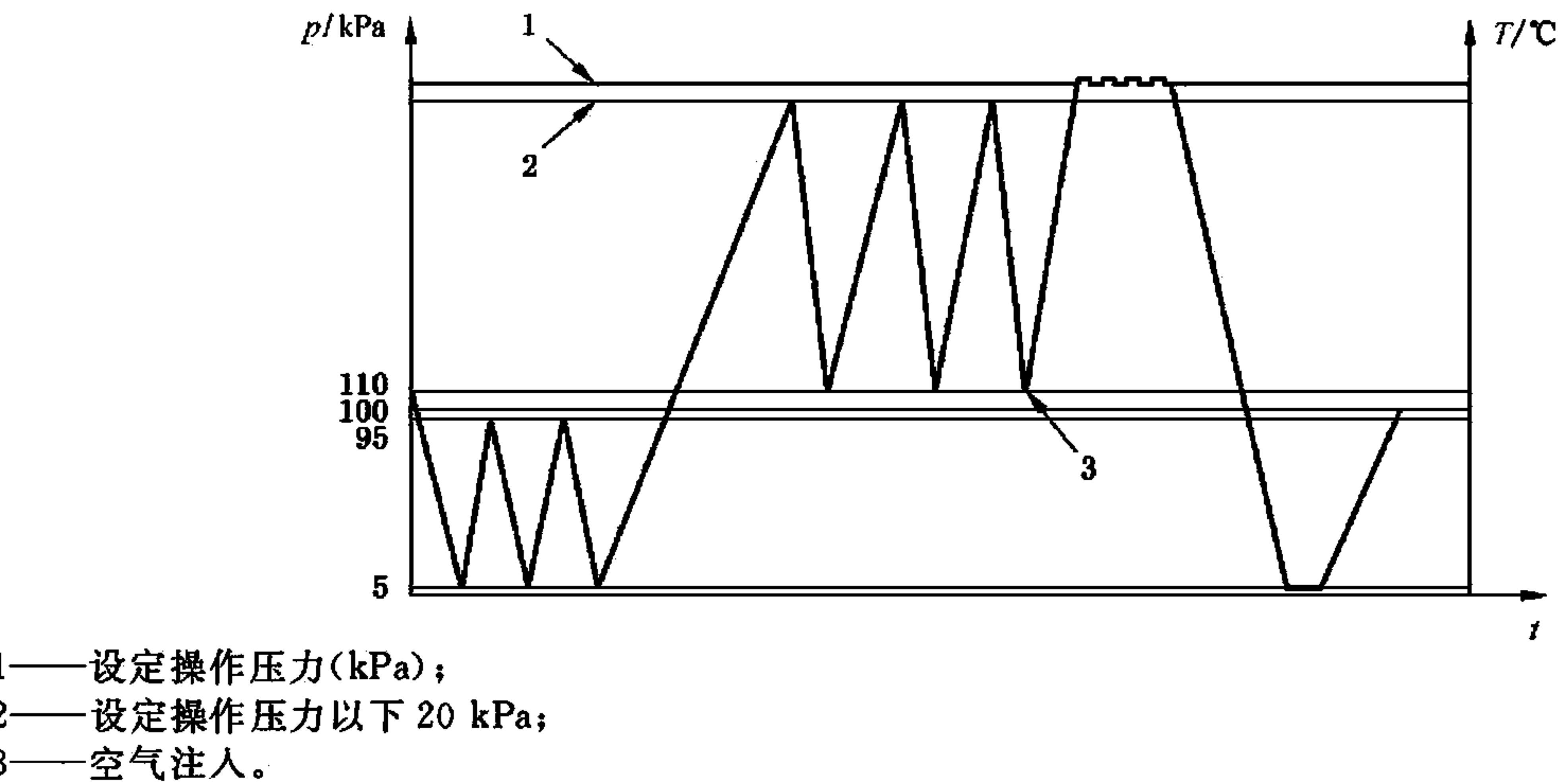
图 B.3 标准测试周期——高大气压排气
