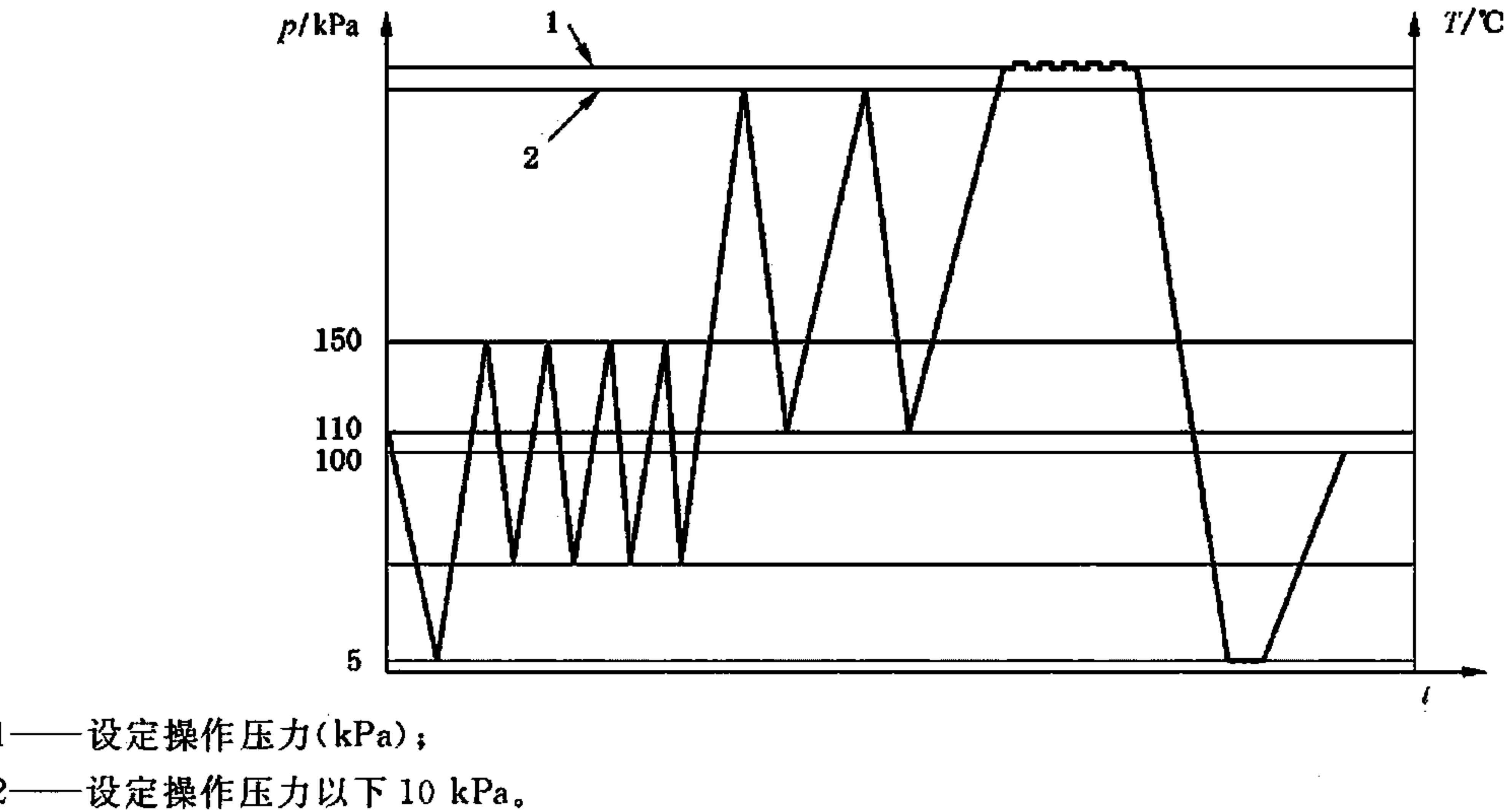
图 B.2 标准测试周期——跨大气压排气
