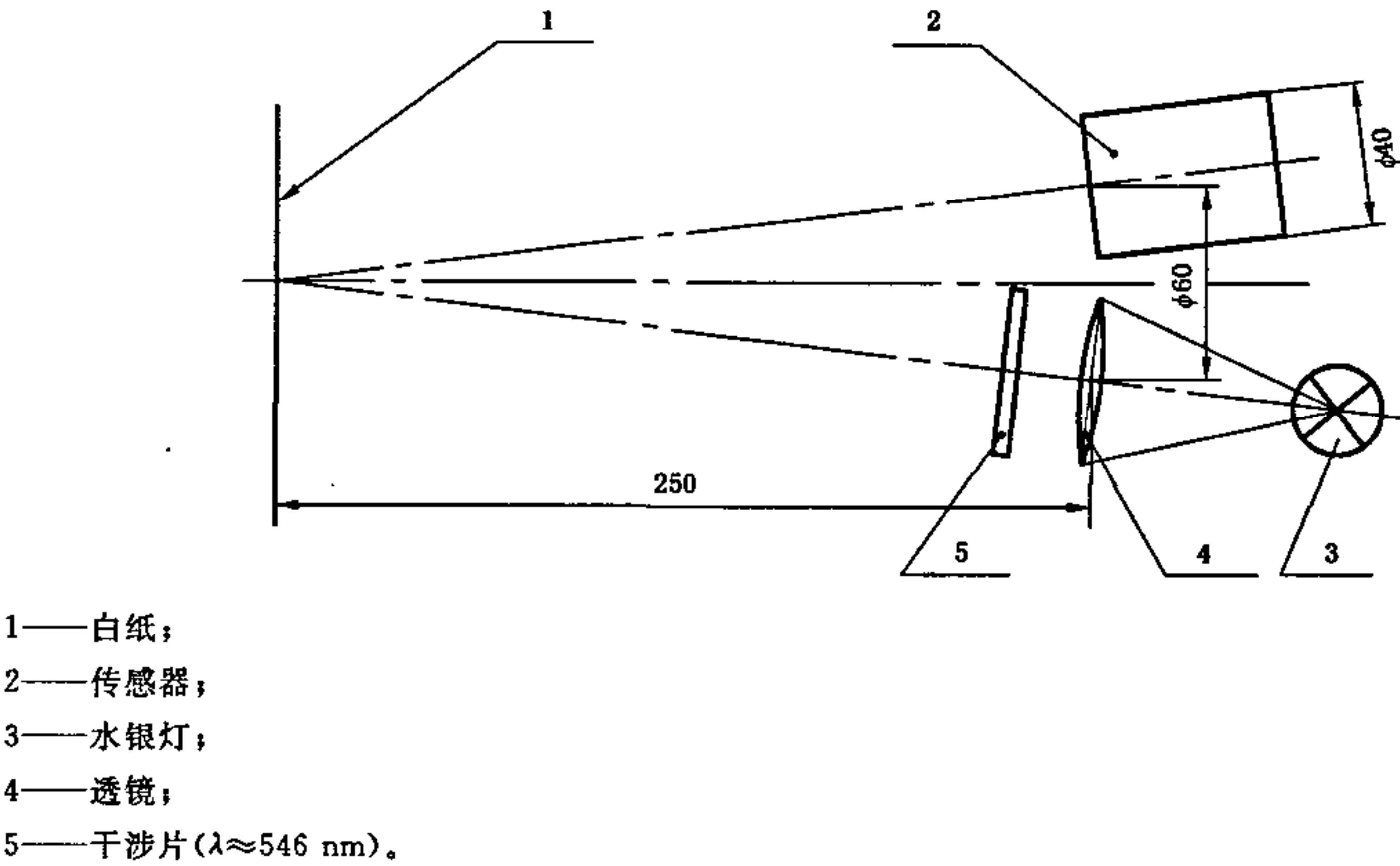
图 9 光电反射计
