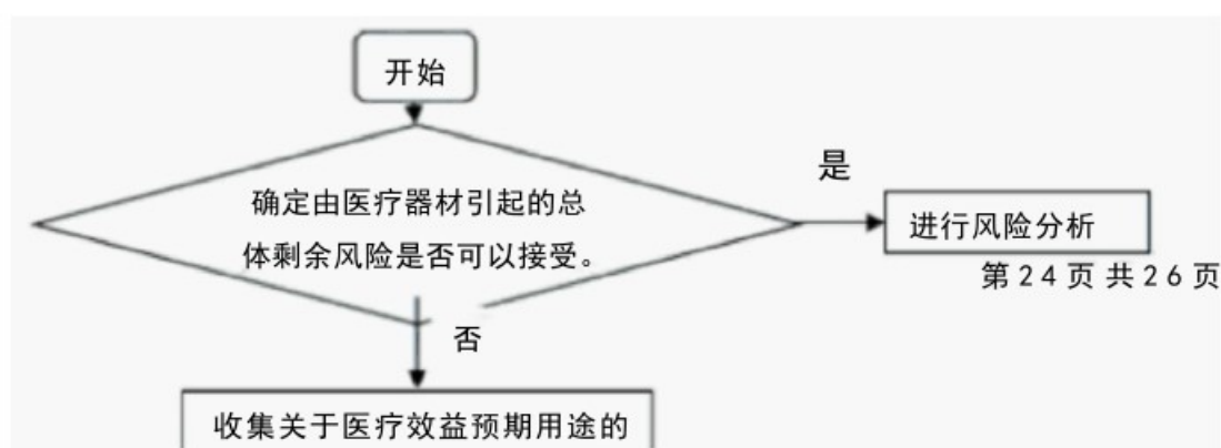
图3评估流程图
