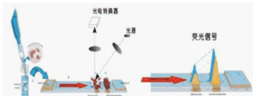
工作原理图
