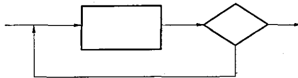
图 17 UNTIL 结构
