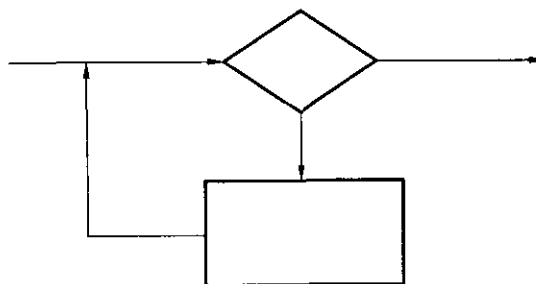
图 18 WHILE 结构
