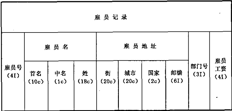
图 7 数据结构图
