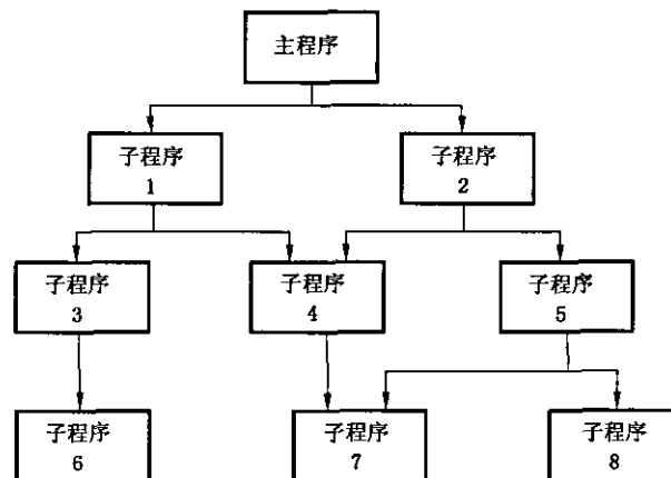
图 4 调用图
