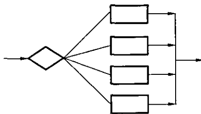
图5 case 结构
