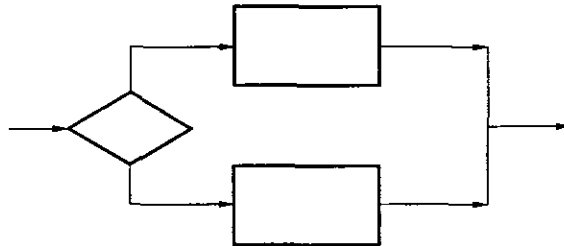
图 13 if-then-else 构造
