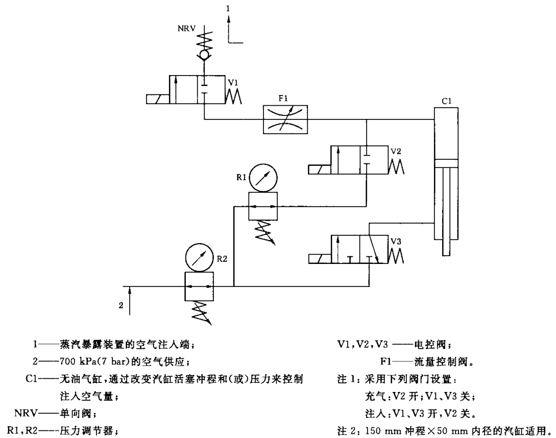
图 J.1 空气注入器设计示意图
