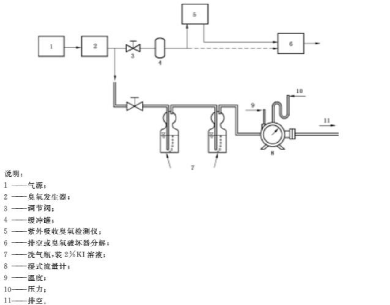
图 B.3 校准系统简图
