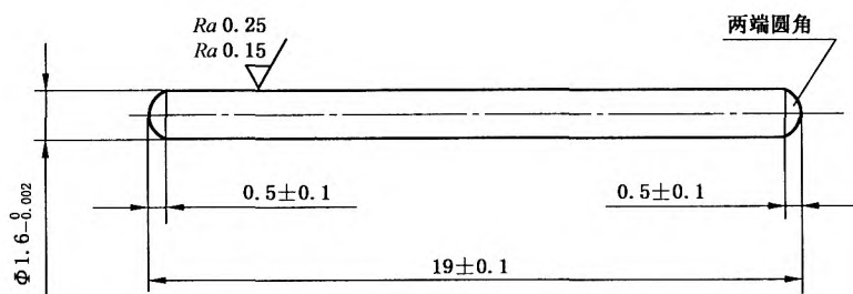
图 2 测试棒
