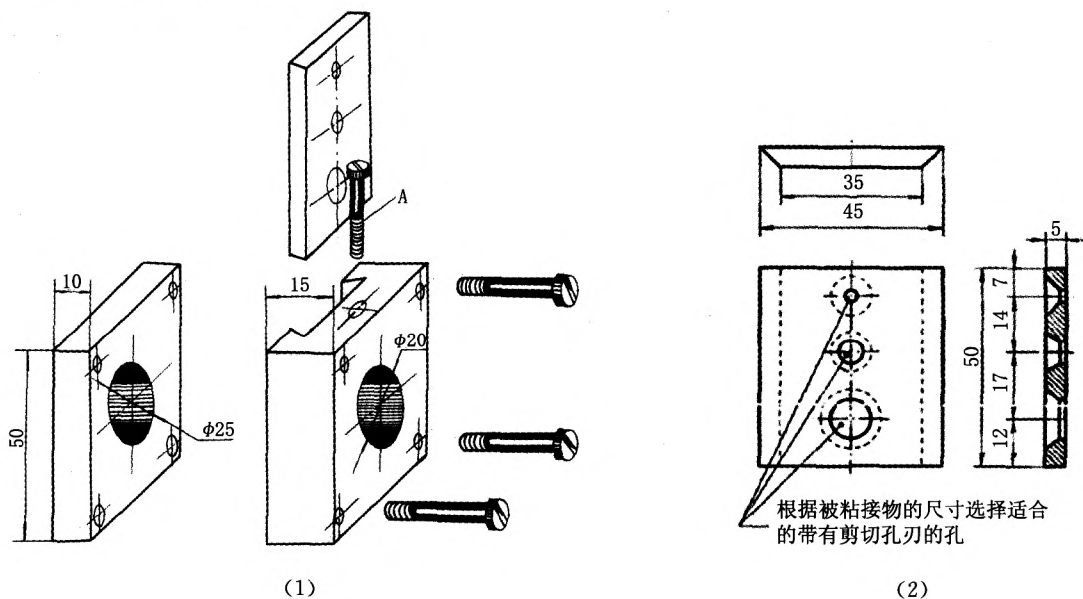
图 D.1 剪切加载装置组合分解示意图
