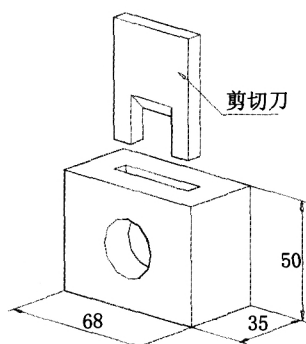
图 C.1 剪切试验器具
