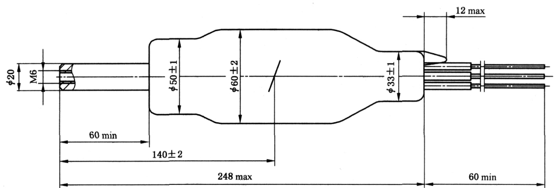
图 A.1 外形图
