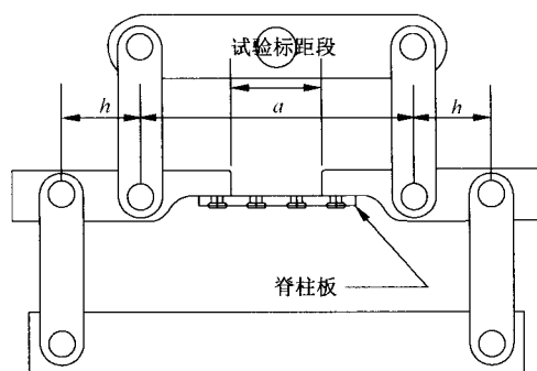
图 3 脊柱板试验装置, R = -1 加载
