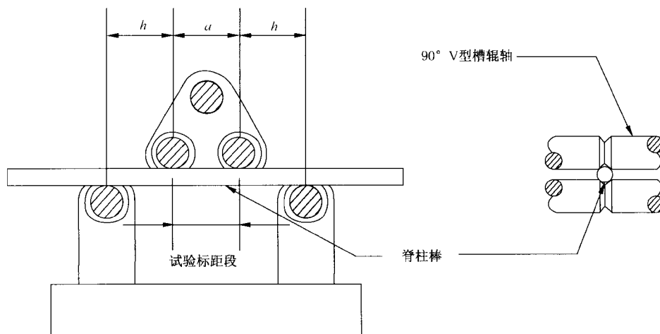
图 2 脊柱棒试验装置
