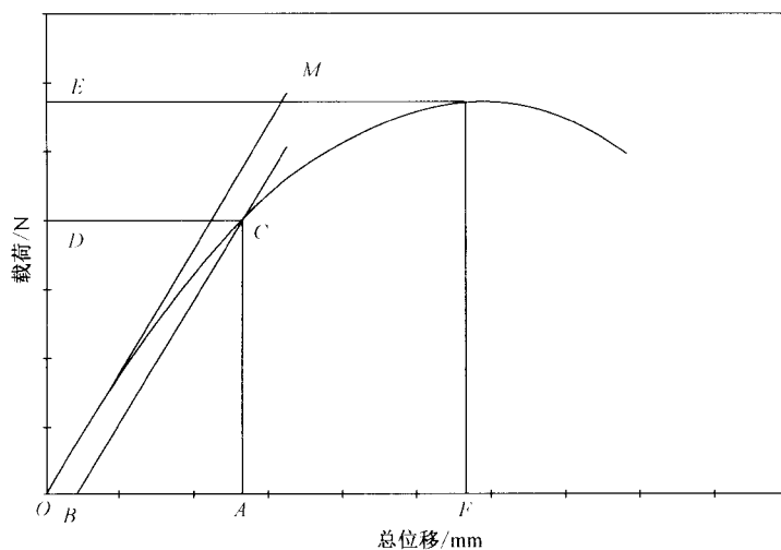
图 4 典型的静态弯曲试验记录
