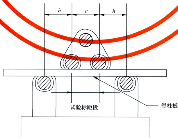
图 1 脊柱板试验装置
