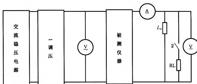
图 2 负载效应试验
