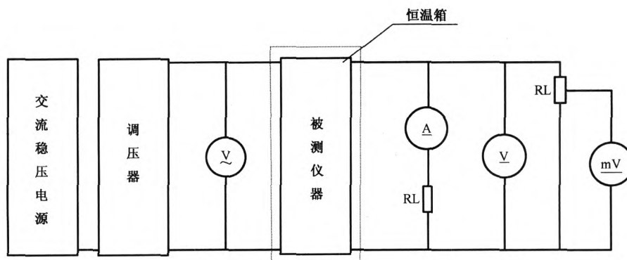
图 4 纹波系数试验
