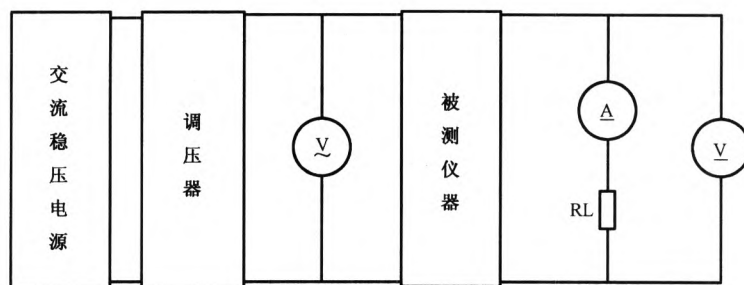
图 1 源电压效应试验
