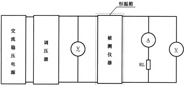
图 3 时间漂移试验和连续工作时间试验
