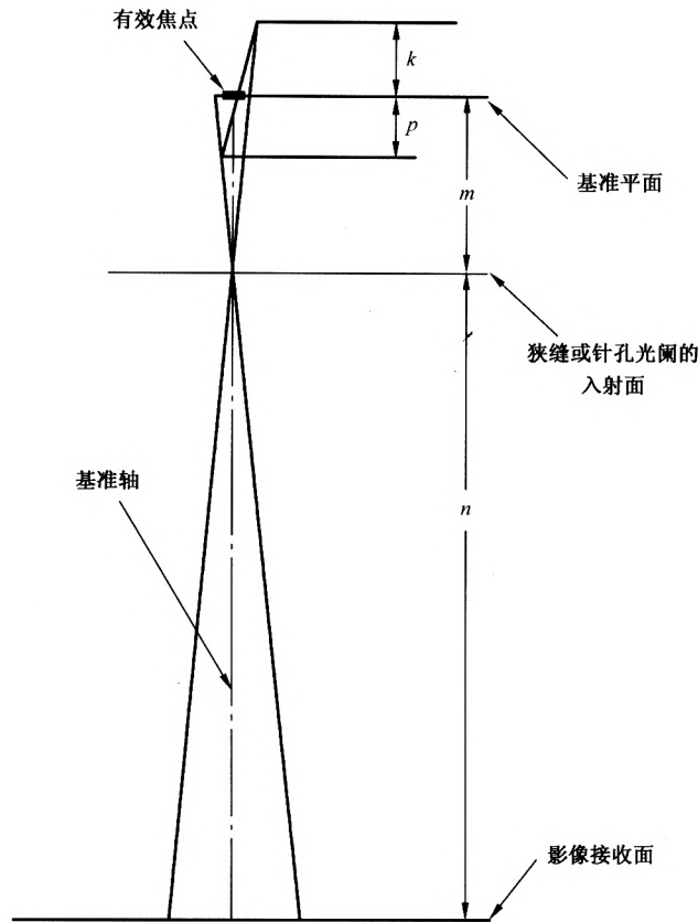
图 4 参照的尺寸和平面
