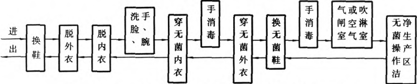
图 D2 人员进出无菌操作洁净生产区的程序图例
